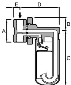
No. 771/C1 萬向接頭 尺寸單位(MM). 最高操作壓力 MOP (KG/CM 2 ). 重量(KG)
