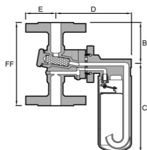
No. 771/C4F 萬向接頭
