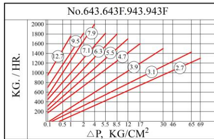
連續排冷凝水量表 公斤/小時 (圓圈為節流孔徑)
