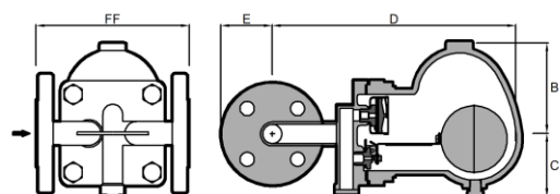
No.FSS2F、FSS5F
