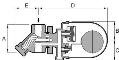
No.F77/C2 尺寸單位(MM). 最高操作壓力 MOP(KG/CM 2 ). 重量(KG)
