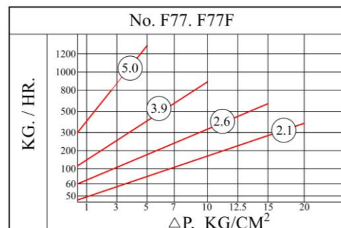
連續排冷凝水量表 公斤/小時
