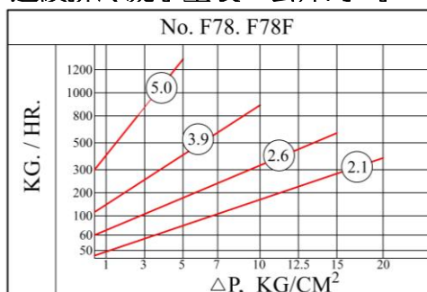
連續排冷凝水量表 公斤/小時
