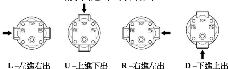
F78 疏水閥進出口方向標示
