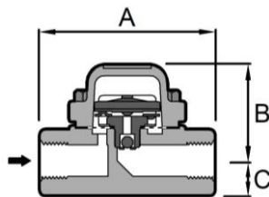
No.S61 尺寸單位(MM). 最高操作壓力 MOP(KG/CM 2 ). 重量(KG)
